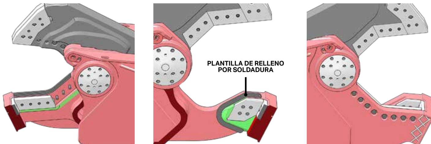
Ubicaciones del relleno por soldadura de la mordaza inferior
