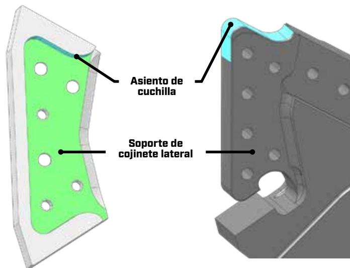
Asiento de la cuchilla y soporte de cojinete lateral FIGURA 33
