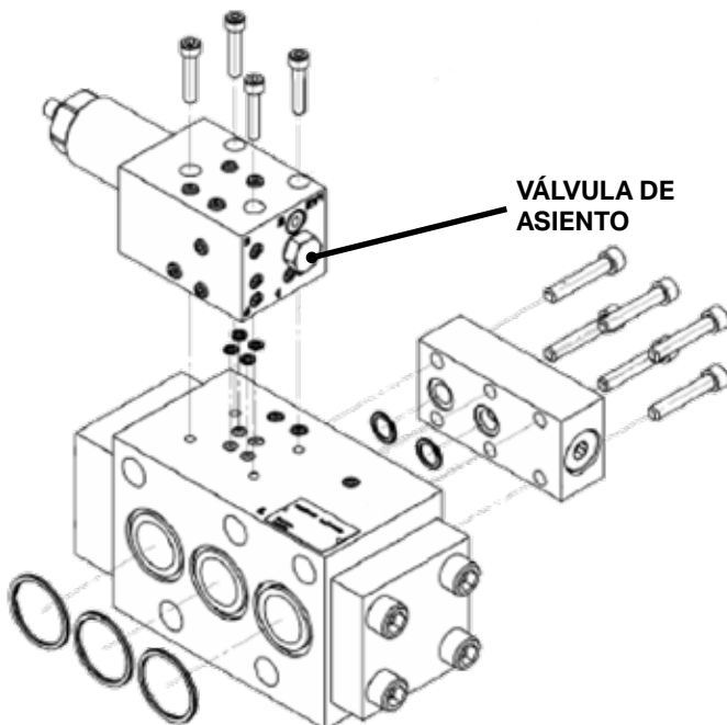
Ubicación de la válvula de asiento
