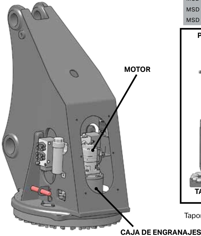
Ubicación de la caja de engranajes planetarios FIGURA 18
