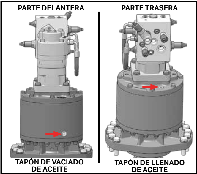
Tapones de vaciado y de llenado de la caja de engranajes FIGURA 19
