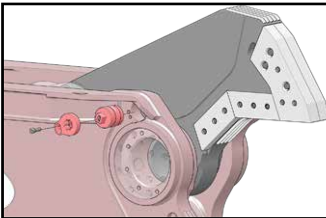
Desmontaje del tornillo deslizante
