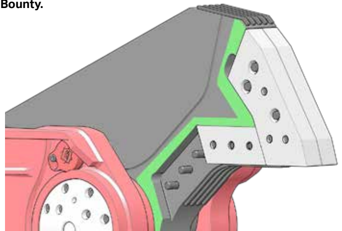
Ejemplo de relleno por soldadura
