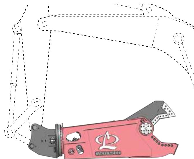
Instalación como tercer miembro FIGURA 10
