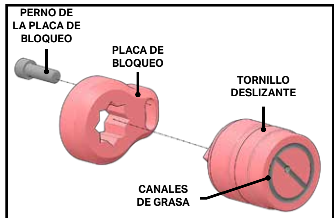
Desmontaje del tornillo deslizante
