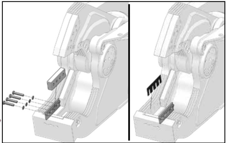
Ajuste con calces de la cuchilla secundaria inferior FIGURA 25
