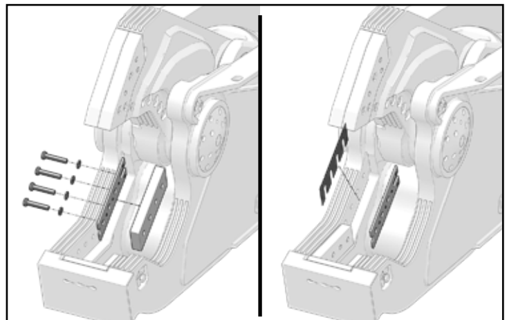
Ajuste con calces de la cuchilla principal inferior FIGURA 27
