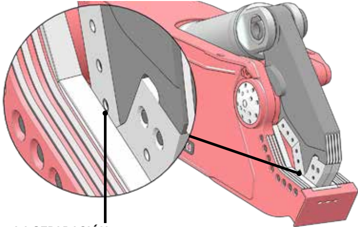
Separación de la cuchilla secundaria FIGURA 24
