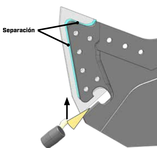
Cuña de la cuchilla y separación FIGURA 32
