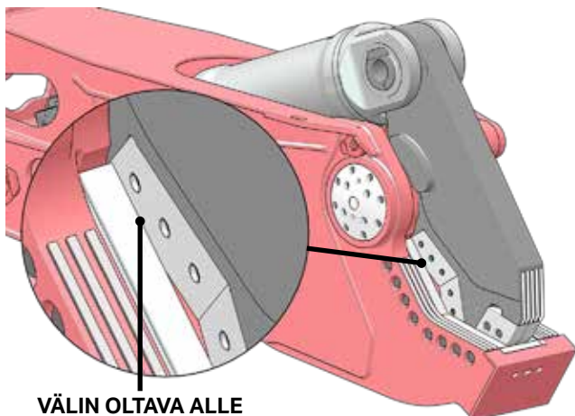
Ensisijaisen terän väli KUVA 26
