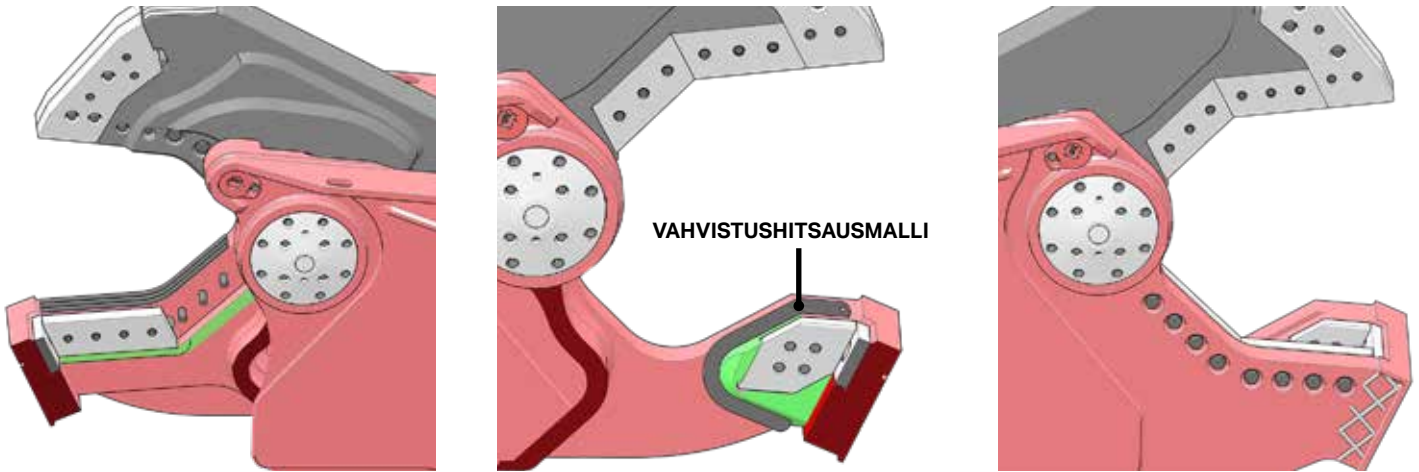
Alaleuan vahvistushitsausten sijainti
