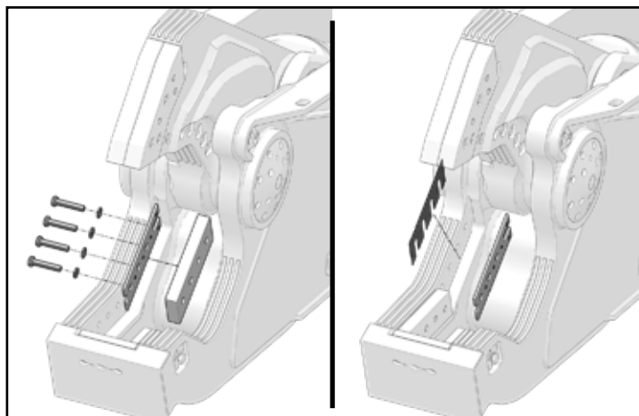
Ensisijaisen alaterän säätö KUVA 27
