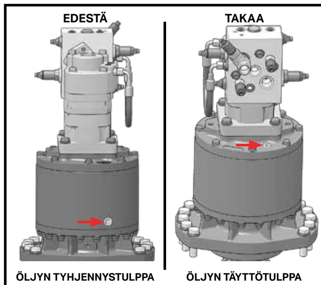
Vaihteiston tyhjennys- ja täyttötulpat KUVA 19
