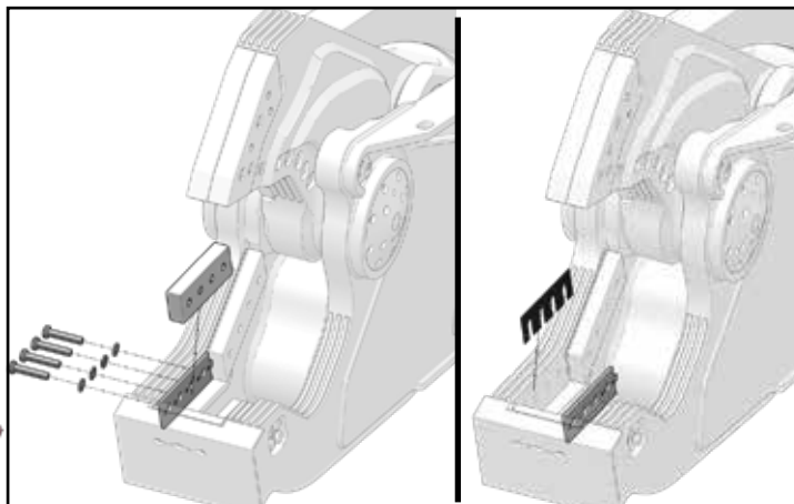
Toissijaisen alaterän säätö KUVA 25
